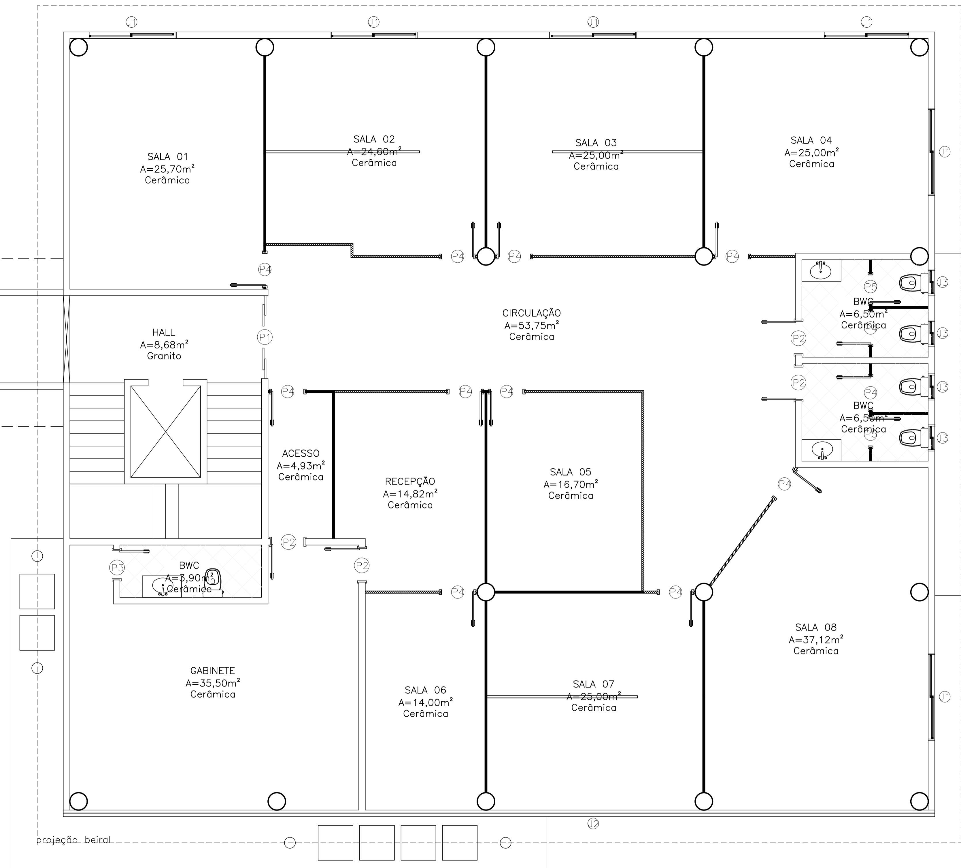
MODULAÇÃO DIVISÓRIAS esc 1:50
