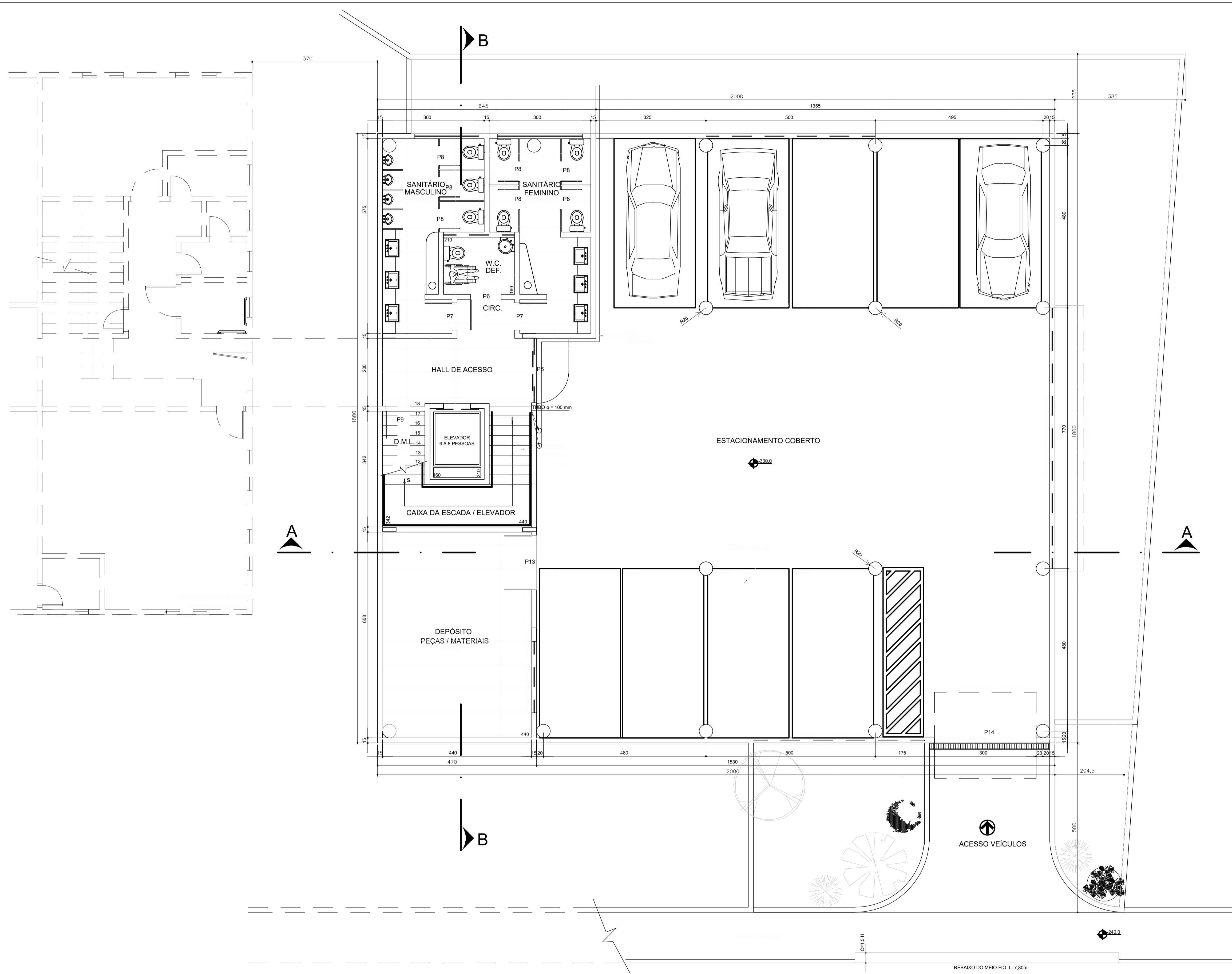
PLANTA BAIXA DO SUBSOLO DO MUSEU ( EXISTENTE ) ESCALA 1:50
