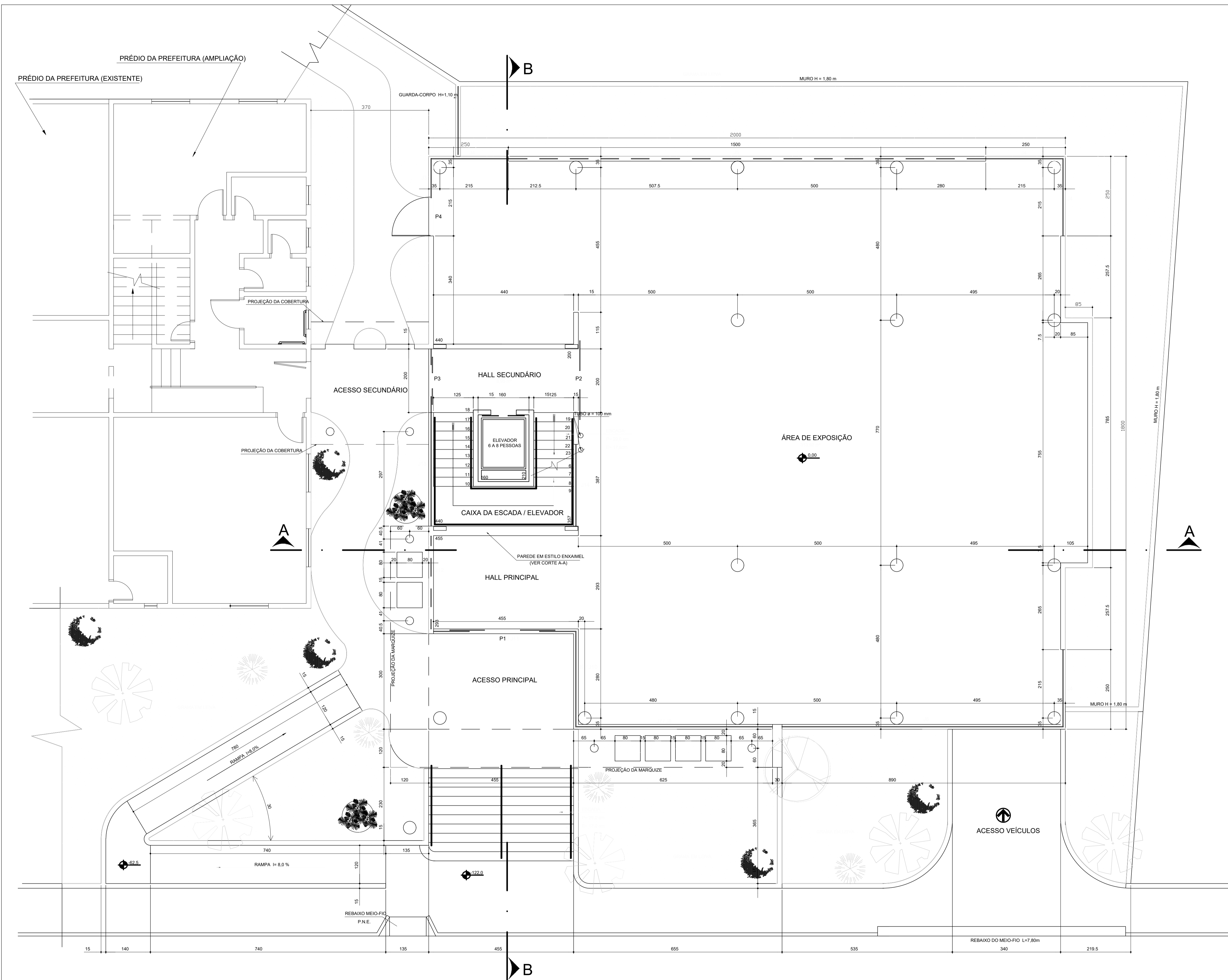
PLANTA BAIXA DO TÉRREO DO MUSEU ( EXISTENTE ) ESCALA 1:50
